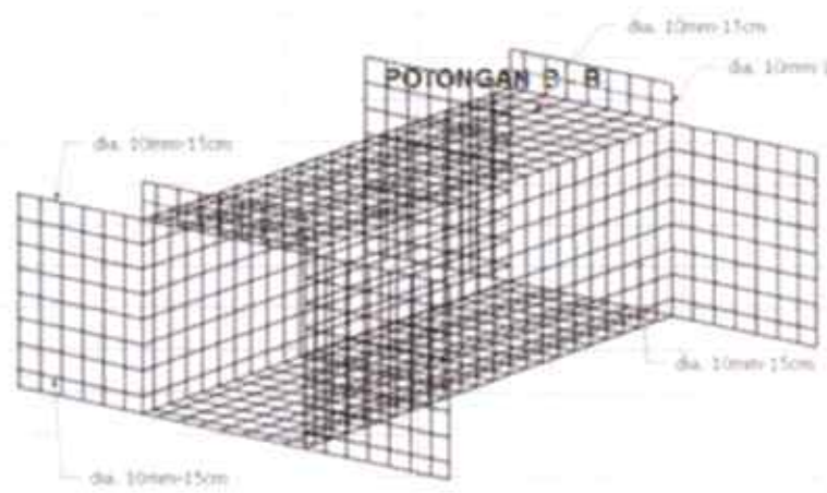
PENULANGAN
